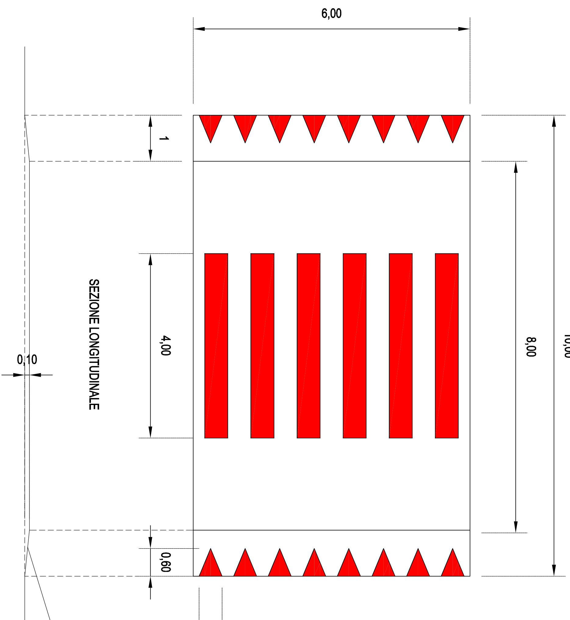
PARTICOLARE PASSAGGIO PEDONALE RIALZATO VIA DELLE AIE - scala 1:50
